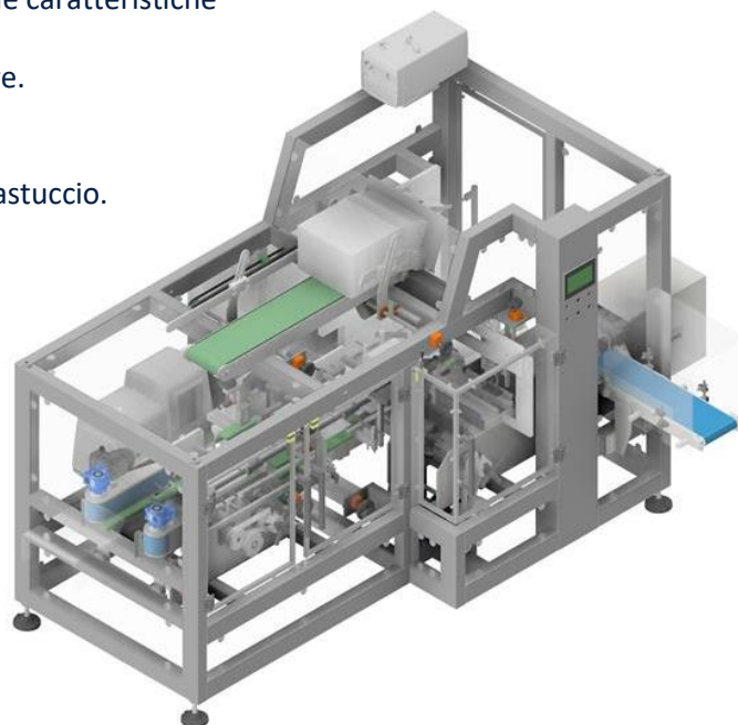
Astucciatrice intermittente mod. AOI040H
