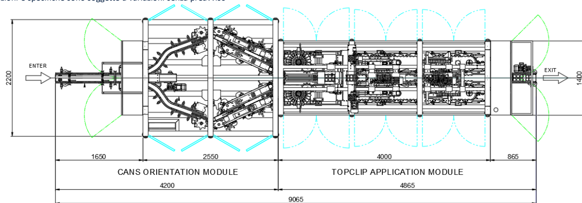
Macchina GreenClip MCC030C con Modulo Orientatore
