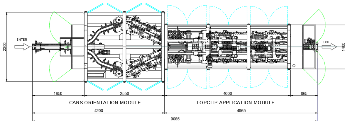
Macchina TopClip MCC030C con Modulo Orientatore
